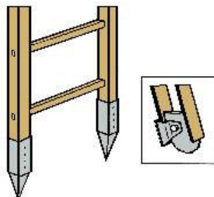
Fig. 6: Tipos de hincas
