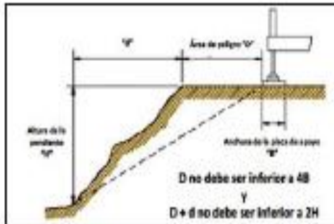
Figura 21. Distancia de seguridad a desniveles.
