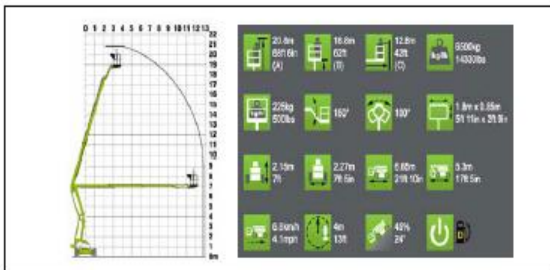
Figura 32. Diagrama de alcance y especificaciones.
